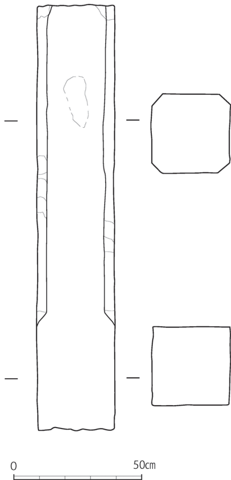
図8 No.9 石柱状石造物 (1:15)
