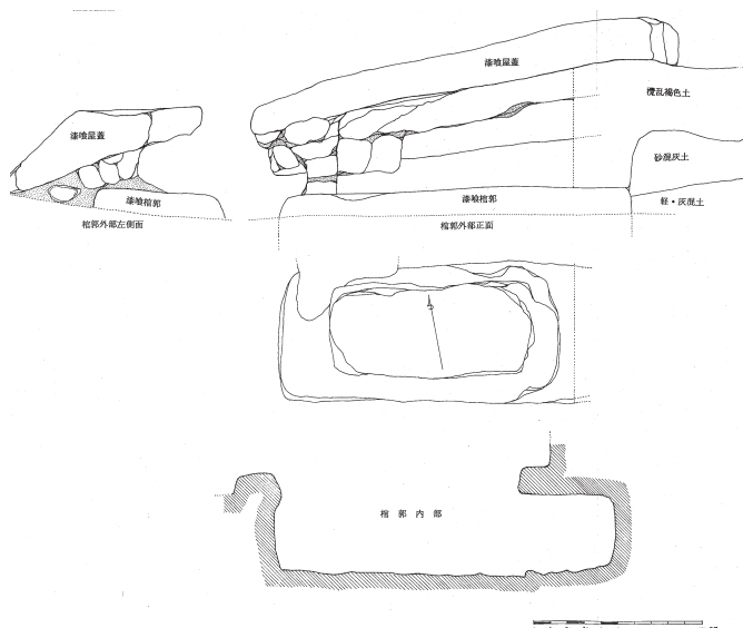
図3 謝振倉墓埋葬施設漆喰郭 (田添 1985 から引用)
