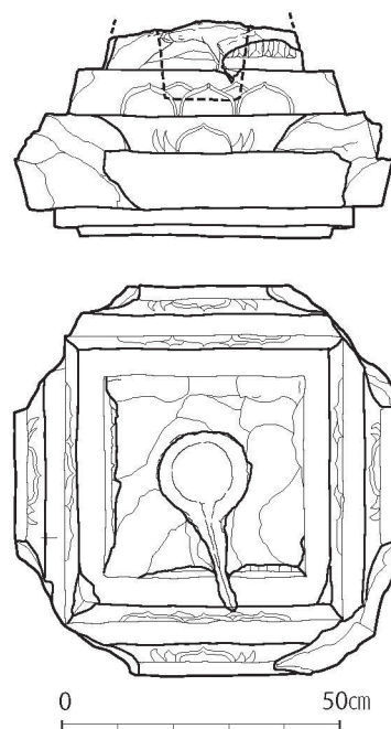
図5 No.3宝篋印塔笠部(1:15)
