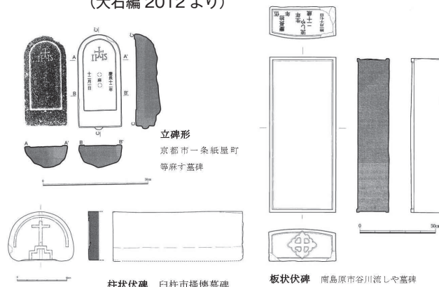
図1 石造キリシタン墓碑の基本3形式 (大石編 2012 より)
