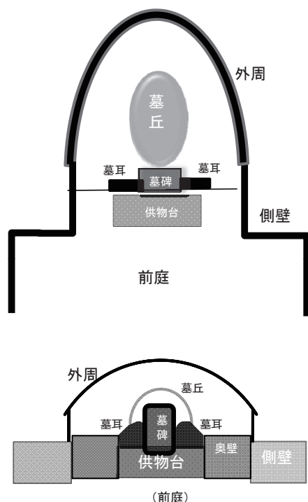
図1 華南様式の唐人墓形態と部位呼称
